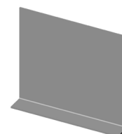
MC Rahmenverlängerung 200 mm (Maß A) Set mit 2 Rahmenverlängerungen, ungebohrt, für Fahrzeuge mit zu geringer Rahmenhöhe (Maß A). Maße (H x B): 200 mm x 230 mm. Rand: 35 mm. 2 Stück Herst.-Nr.: 227-1021 Art-Nr. 115/119
