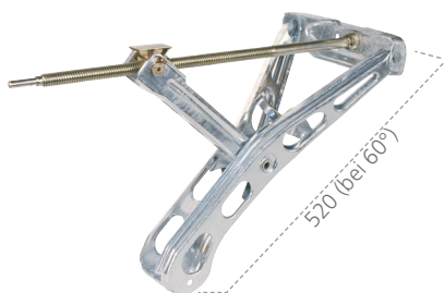
Steckstützen Premium 1200 L Tragfähigkeit: 1250 kg; zul. Gewicht: 2500 kg; Gewicht: 5 kg Herst.-Nr.: 1224510 Art-Nr. 120/007
