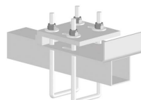
MC Befestigungssatz Eriba Troll Set mit 2 Adaptersätzen für Hymer Eriba Troll-Modelle mit Vierkantrohr-Rahmen und L-Profil. 2 Stück Herst.-Nr.: 227-1036 Art-Nr. 115/096
