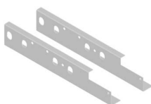
MC Befestigungssatz 3.6 Reserverad für Verlegung des AL-KO-Reserveradträgers um 90 mm nach hinten. 2 Stück Herst.-Nr.: 227-1145 Art-Nr. 115/093
